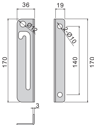
B-1083-30-L B-83-30-L
