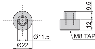
B-1083-M8 B-83-M8
