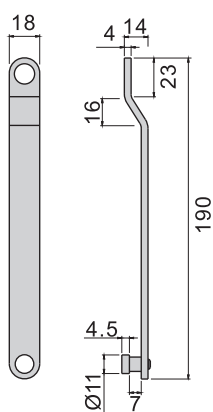
B-1083-S2 B-83-S2
