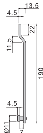
B-1083-S3 B-83-S3
