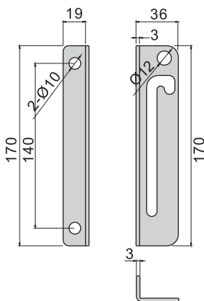
B-1083-30-R B-83-30-R
